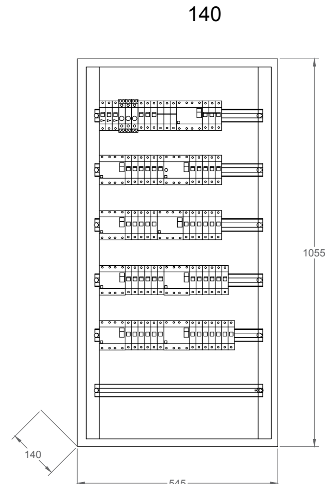
Obudowa modułowa IP30 Gł. [mm] 140
