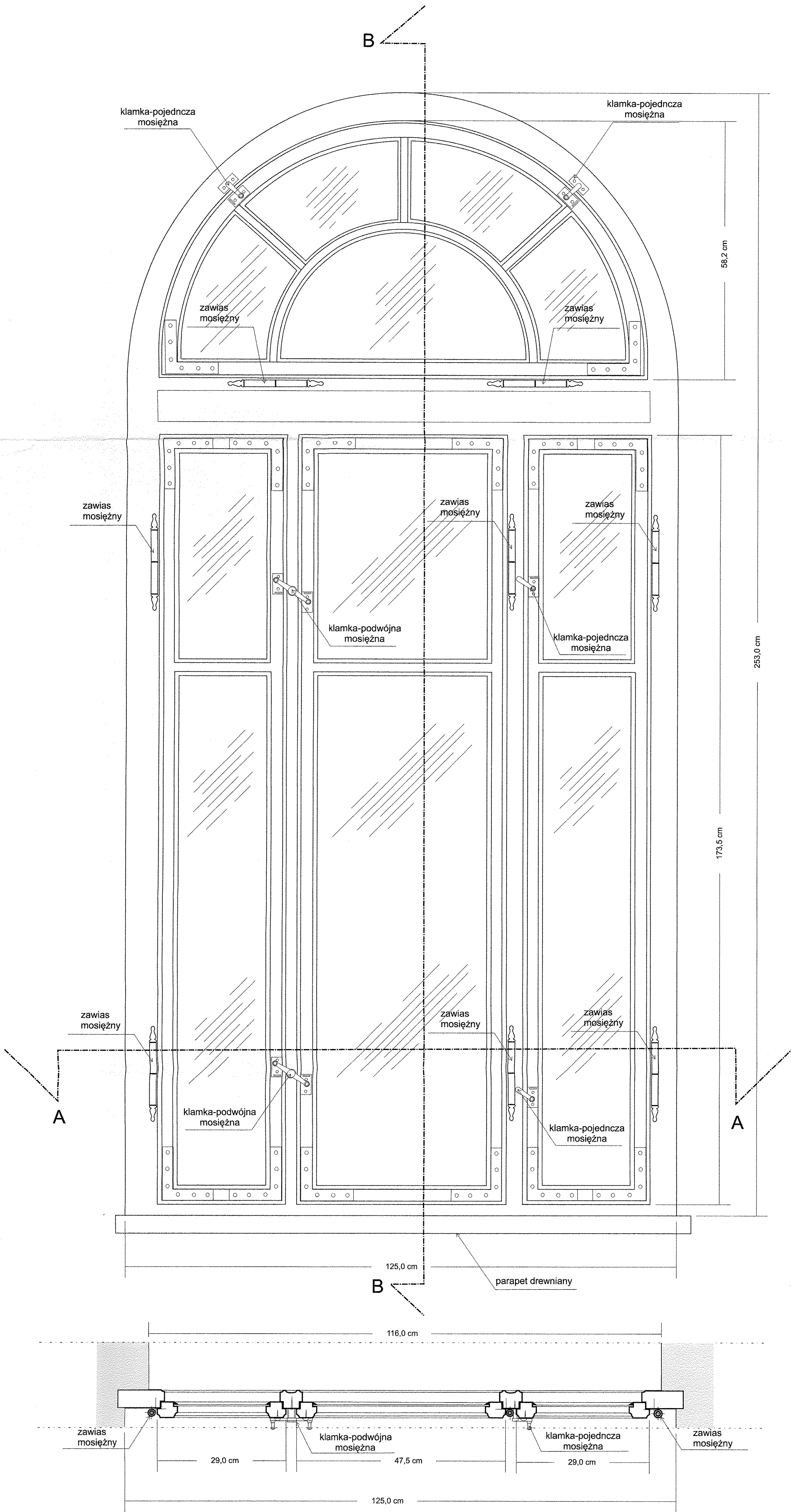
Przekrój A-A
